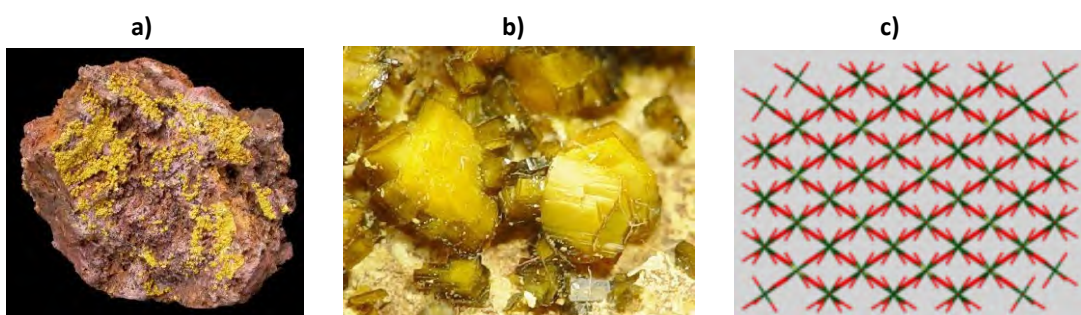
Rys. 3. Mineral soddyit: (a) skała, (b) wygląd kryształów, (c) struktura krystaliczna [Źródło: https://en.wikipedia.org/wiki/Frederick_Soddy ; https://de.wikipedia.org/wiki/Soddyit#/media/Datei:Soddyite-Swamboite-180982.jpg https://de.wikipedia.org/wiki/Soddyit#/media/Datei:Soddyite_-_packing_c_axis_(a_up,_b_right).png ]
